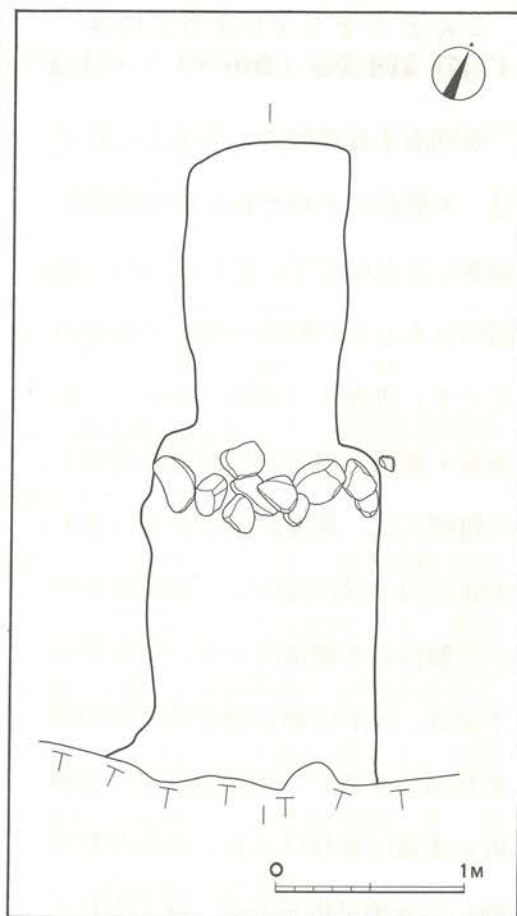
第6図 南第22号横穴平面図
